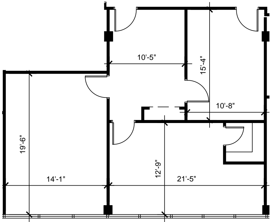
1 FLOOR PLAN SCALE: 1/8" = 1'-0"
